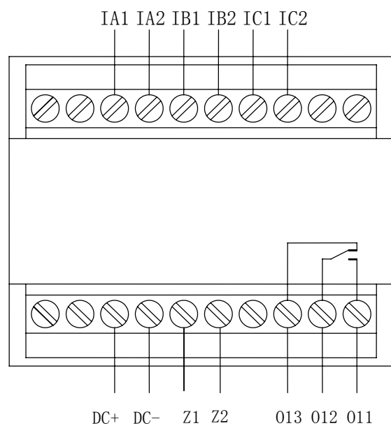
AMDG-□/A011 系列保护器主单元端子图
