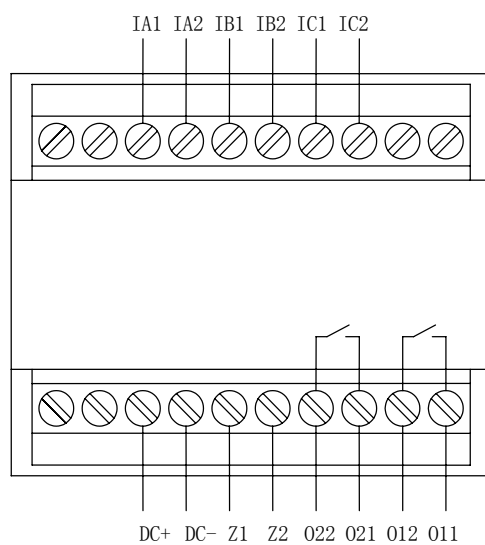
AMDG-□/A013 系列保护器主单元端子图
