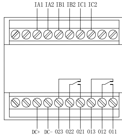
AMDG-□/A002 系列保护器主单元端子图
