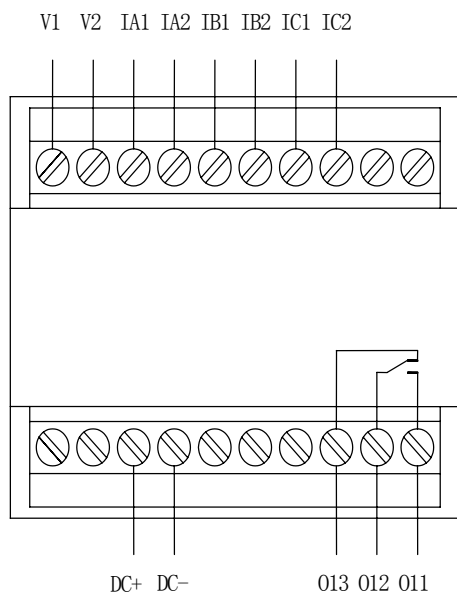
AMDG-□/A0□1 系列保护器主单元端子图
