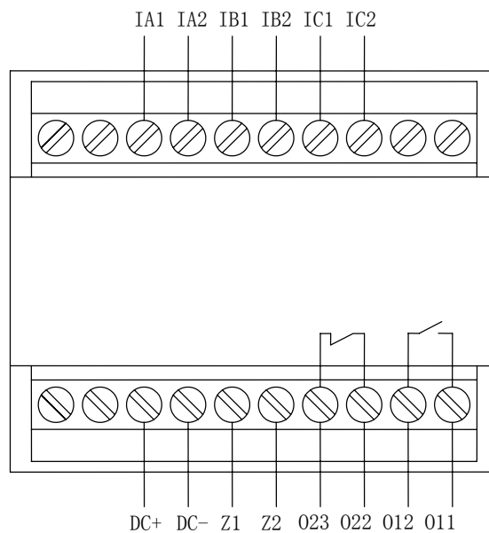
AMDG-□/A014 系列保护器主单元端子图
