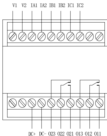
AMDG-□/A0□2 系列保护器主单元端子图
