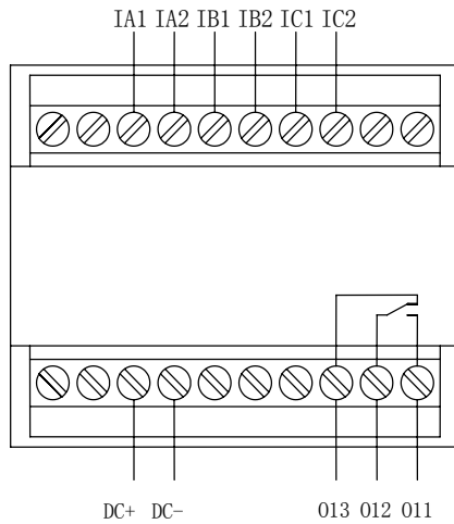
AMDG-□/A001 系列保护器主单元端子图
