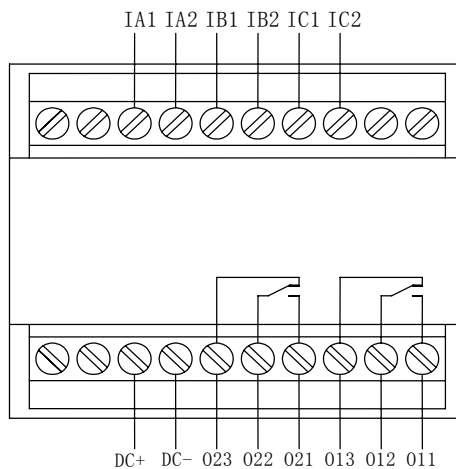
AMDG-□/B002 系列保护器主单元端子图
