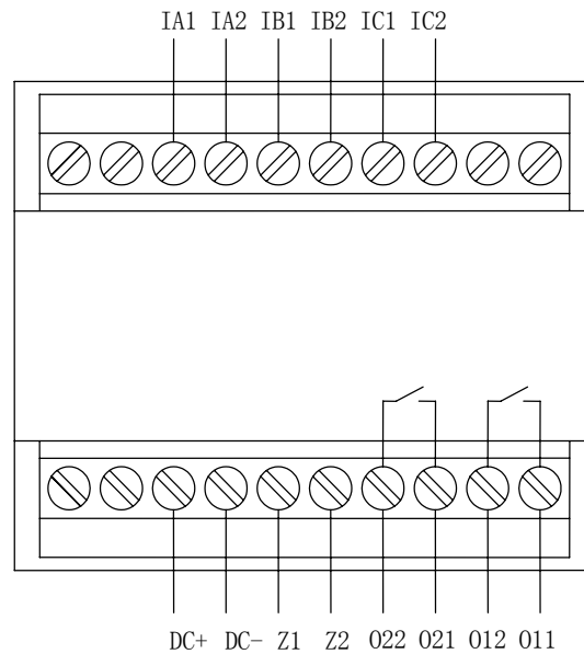
AMDG-□/B013 系列保护器主单元端子图
