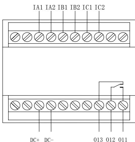
AMDG-□/B001 系列保护器主单元端子图
