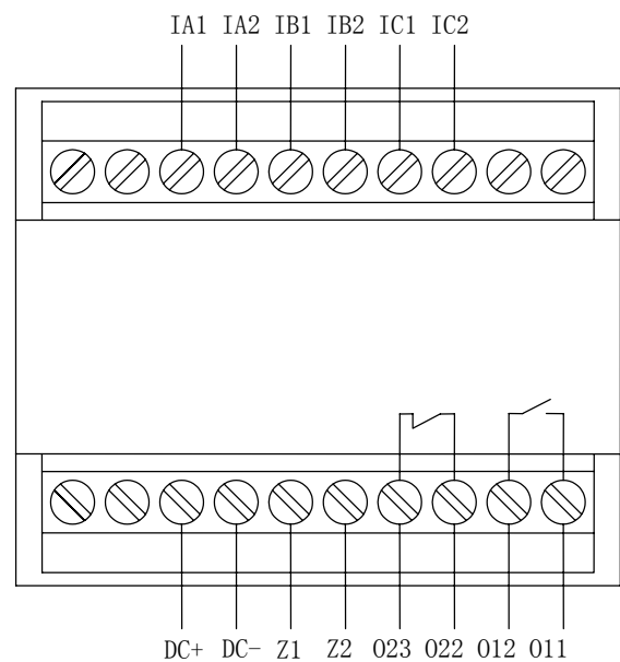
AMDG-□/B014 系列保护器主单元端子图
