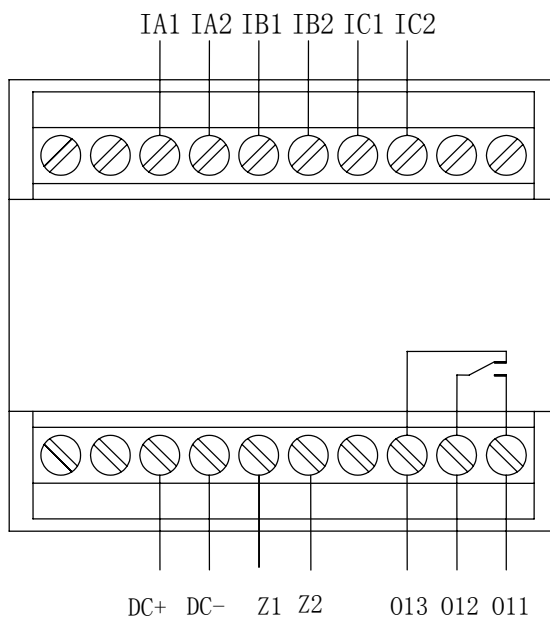
AMDG-□/B011 系列保护器主单元端子图
