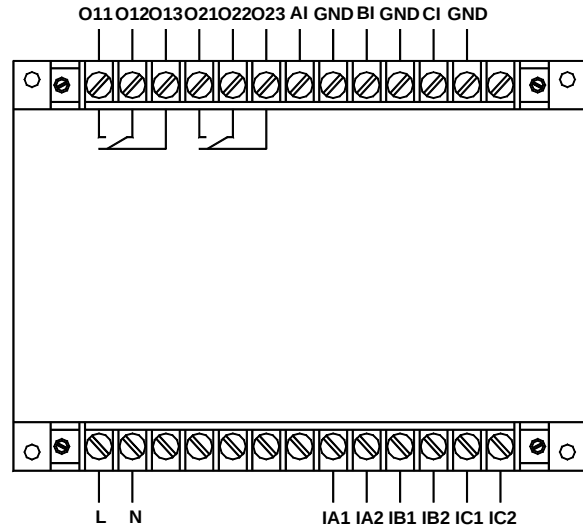
AMDG-□/C102 系列保护器主单元端子图
