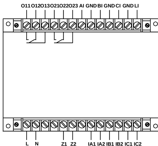
AMDG-□/□/□ 系列保护器主单元端子图
