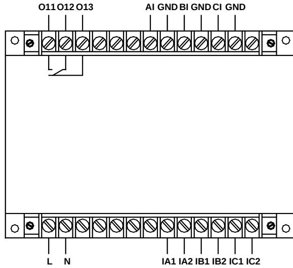
AMDG-□/C101 系列保护器主单元端子图
