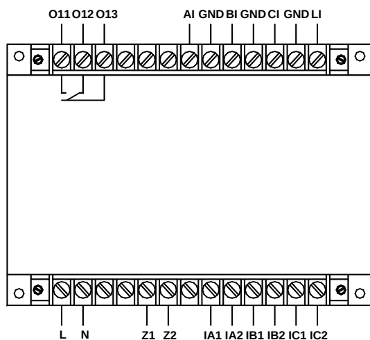
AMDG-□/□/□ 系列保护器主单元端子图
