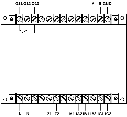
AMDG-□/C211 系列保护器主单元端子图
