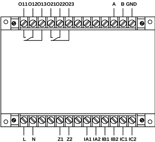
AMDG-□/C212 系列保护器主单元端子图
