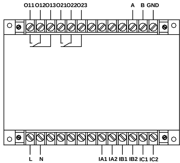
AMDG-□/C202 系列保护器主单元端子图
