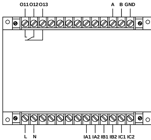
AMDG-□/C201 系列保护器主单元端子图
