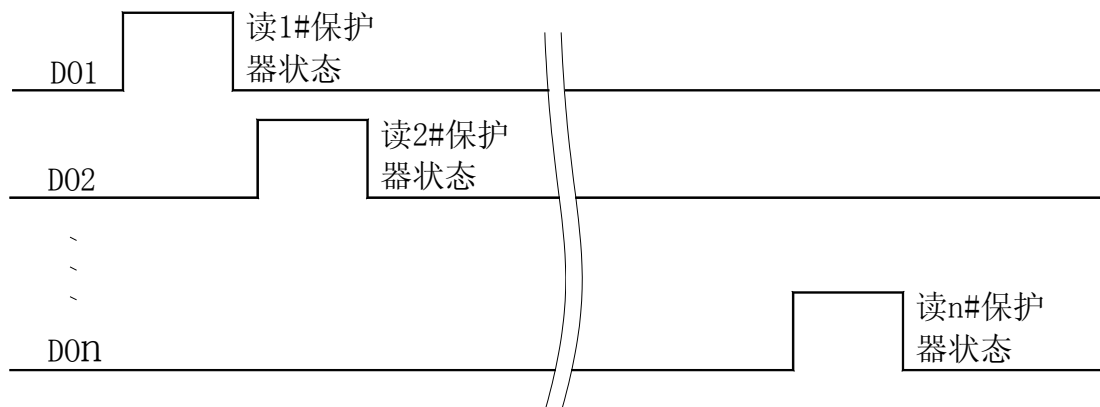
PLC 读取多台 AMDG-□/C6 系列电动机保护器时序图
