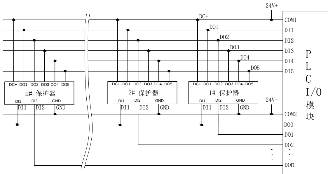
PLC 读取多台 AMDG-□/C6 系列电动机保护器电气原理图
