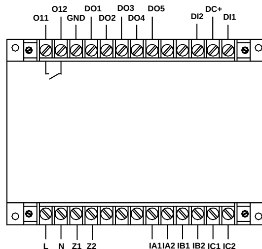
AMDG-□/C611 系列保护器主单元端子图
