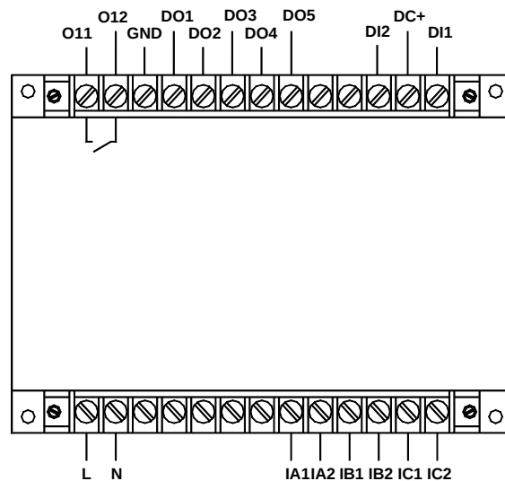
AMDG-□/C601 系列保护器主单元端子图
