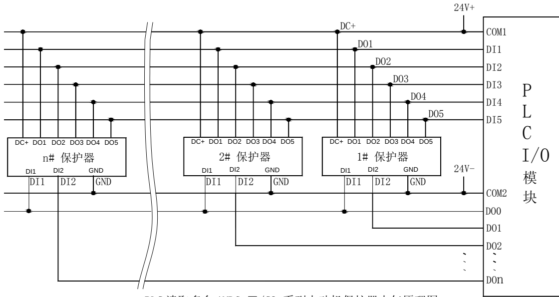
PLC 读取多台 AMDG-□/C8 系列电动机保护器电气原理图
