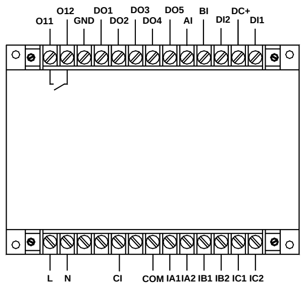
AMDG-□/C801 系列保护器主单元端子图
