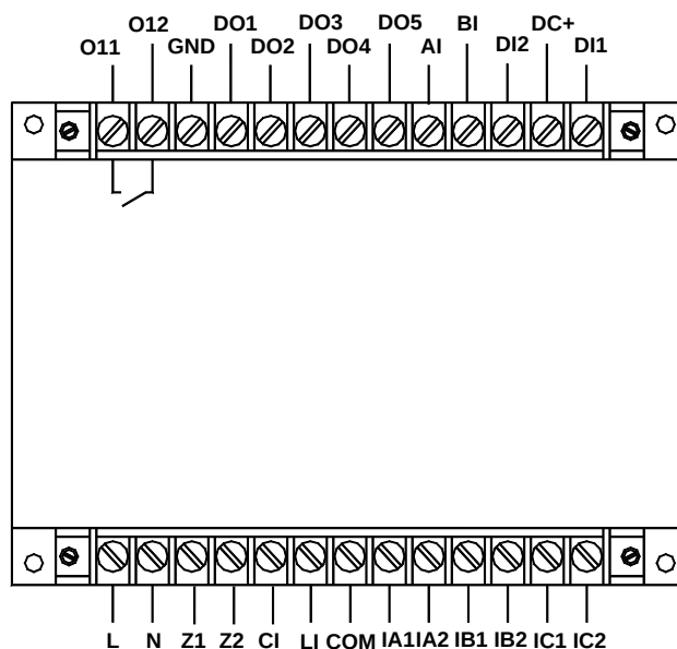
AMDG-□/C811 系列保护器主单元端子图
