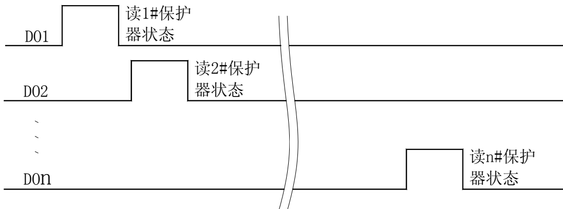
PLC 读取多台 AMDG-□/C8 系列电动机保护器时序图
