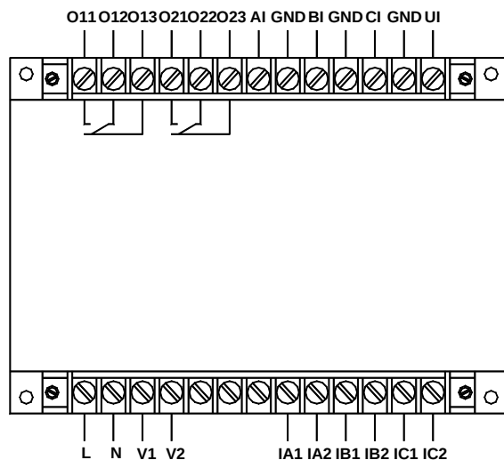
AMDG-□/D102 系列保护器主单元端子图
