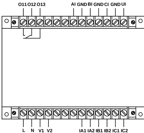
AMDG-□/D101 系列保护器主单元端子图
