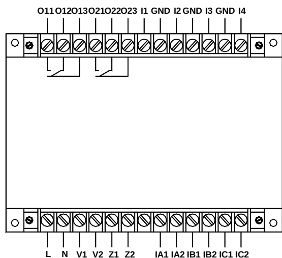
AMDG-□/D112 系列保护器主单元端子图
