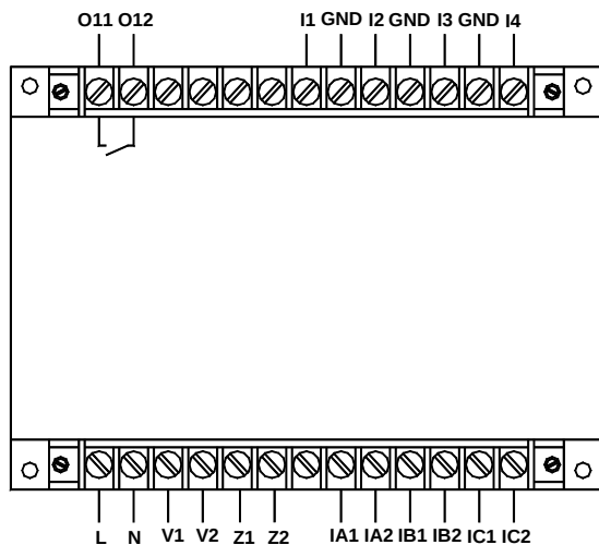
AMDG-□/D111 系列保护器主单元端子图
