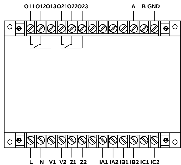
AMDG-□/D212 系列保护器主单元端子图
