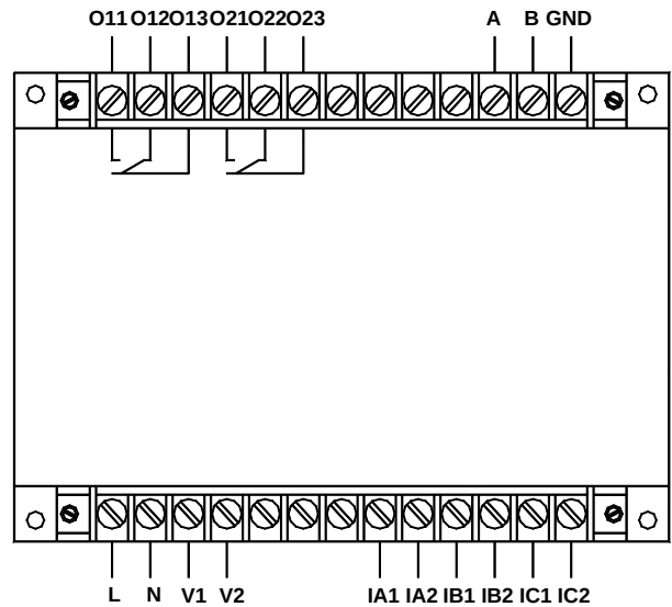
AMDG-□/D202 系列保护器主单元端子图
