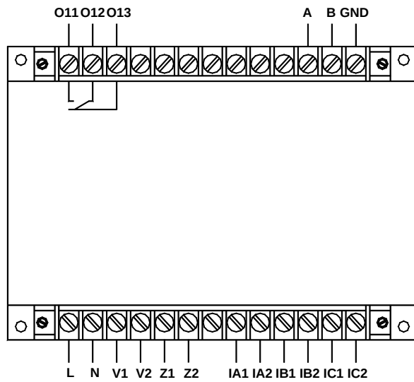
AMDG-□/D211 系列保护器主单元端子图
