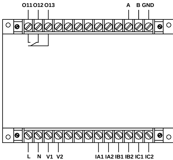
AMDG-□/D201 系列保护器主单元端子图
