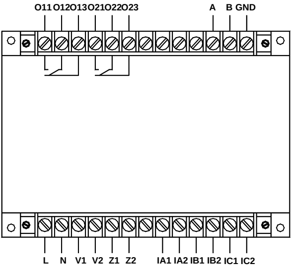
AMDG-□/D312 系列保护器主单元端子图
