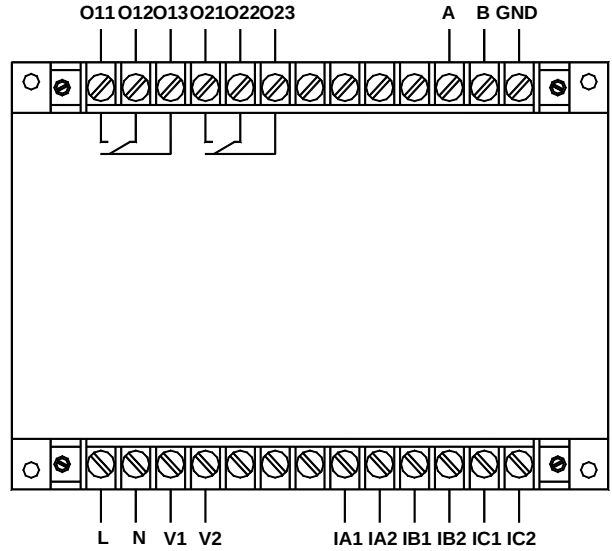
AMDG-□/D302 系列保护器主单元端子图
