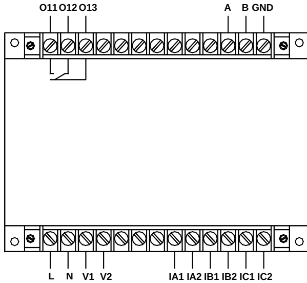
AMDG-□/D301 系列保护器主单元端子图
