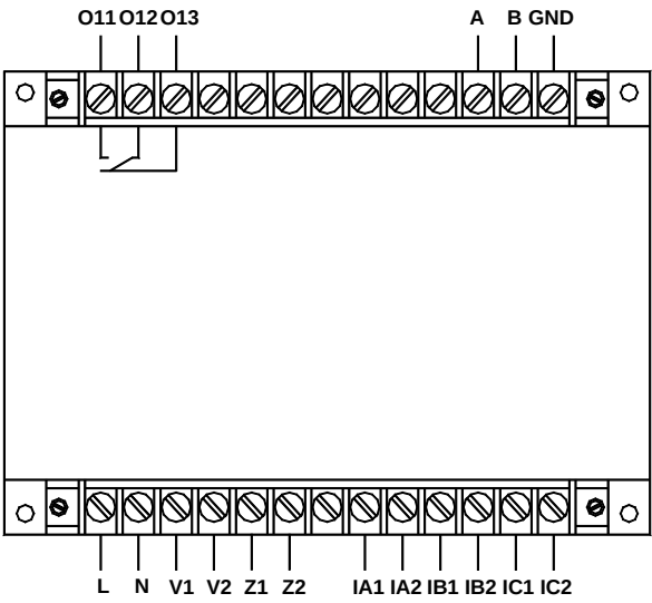
AMDG-□/D311 系列保护器主单元端子图
