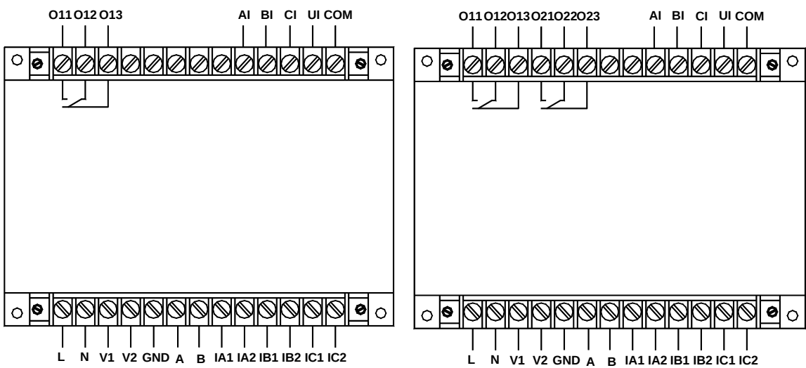
AMDG-□/D4□1 系列保护器主单元端子图
