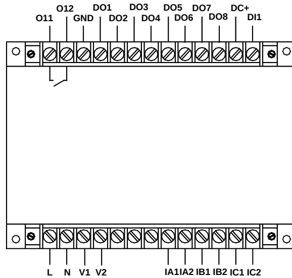
AMDG-□/D5□1 系列保护器主单元端子图
