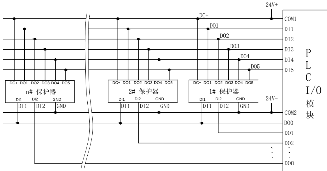
PLC 读取多台 AMDG-□/D6 系列电动机保护器电气原理图
