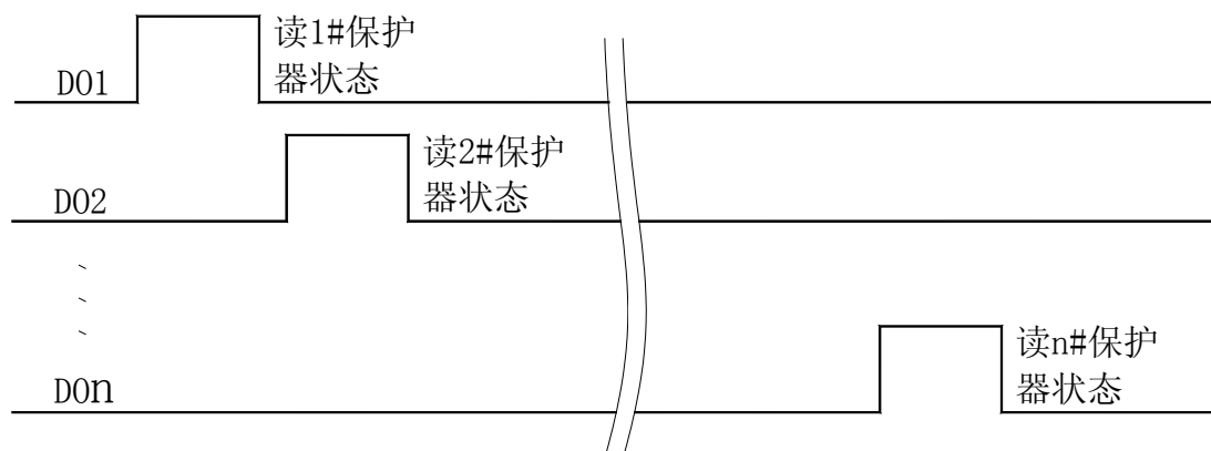
PLC 读取多台 AMDG-□/D6 系列电动机保护器时序图
