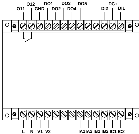
AMDG-□/D6□1 系列保护器主单元端子图
