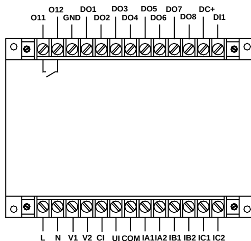
AMDG-□/D7□1 系列保护器主单元端子图
