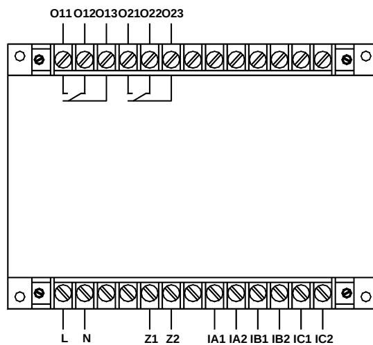
AMDG-X/E012 系列保护器主单元端子图
