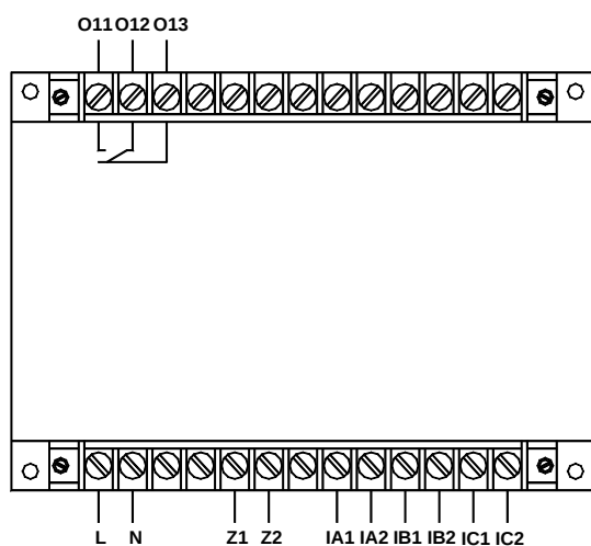
AMDG-X/E011 系列保护器主单元端子图
