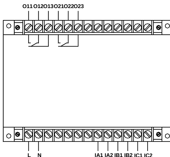
AMDG-X/E002 系列保护器主单元端子图
