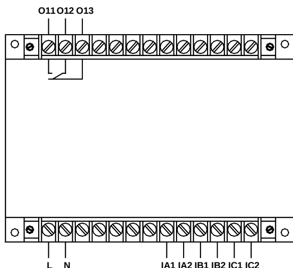
AMDG-X/E001 系列保护器主单元端子图
