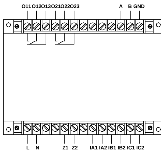
AMDG-X/E212 系列保护器主单元端子图
