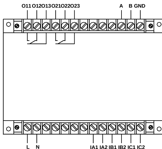
AMDG-X/E202 系列保护器主单元端子图
