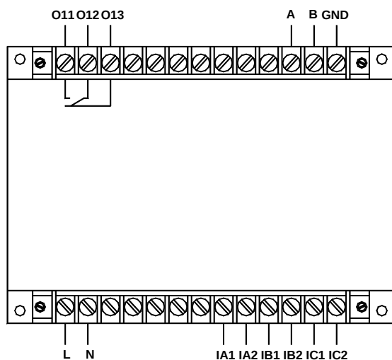
AMDG-X/E201 系列保护器主单元端子图
