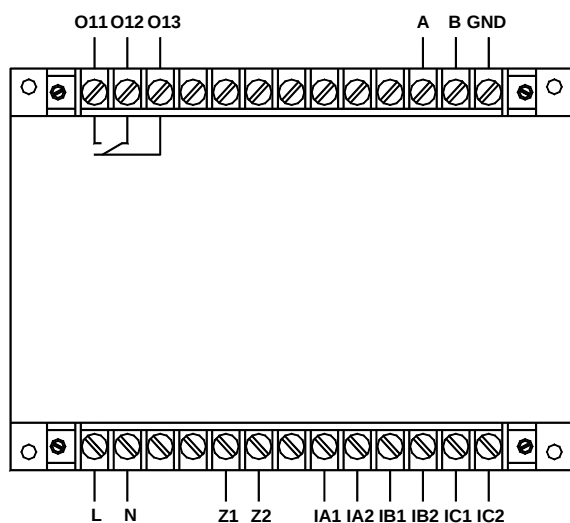
AMDG-X/E211 系列保护器主单元端子图
