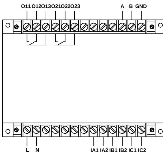
AMDG-X/E302 系列保护器主单元端子图
