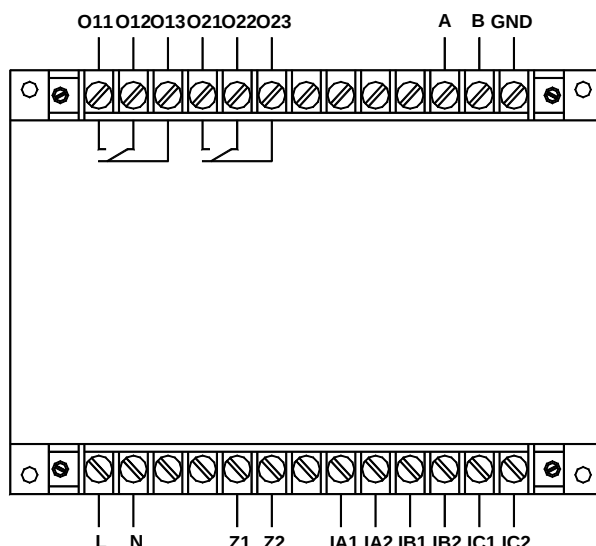
AMDG-X/E312 系列保护器主单元端子图
