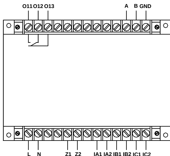
AMDG-X/E311 系列保护器主单元端子图
