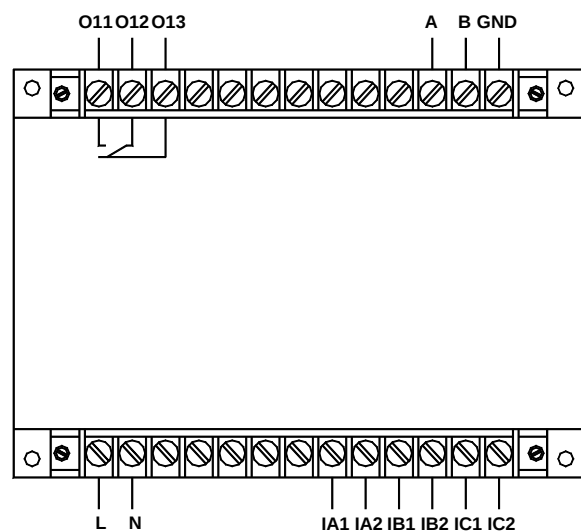
AMDG-X/E301 系列保护器主单元端子图
