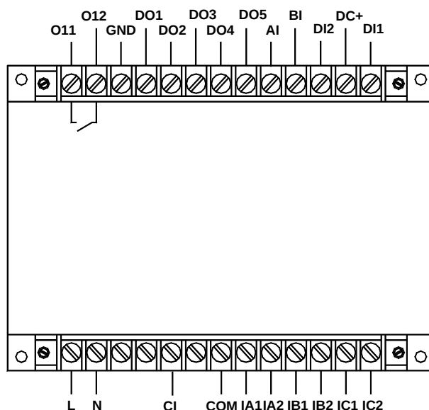
AMDG-X/E801 系列保护器主单元端子图
