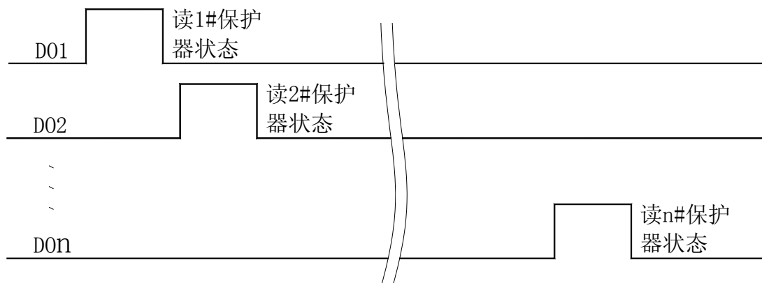
PLC 读取多台 AMDG-X/E8 系列电动机保护器时序图
