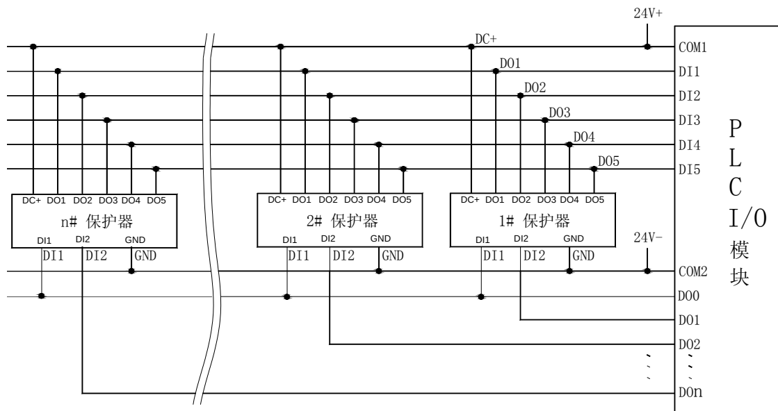
PLC 读取多台 AMDG-X/E8 系列电动机保护器电气原理图
