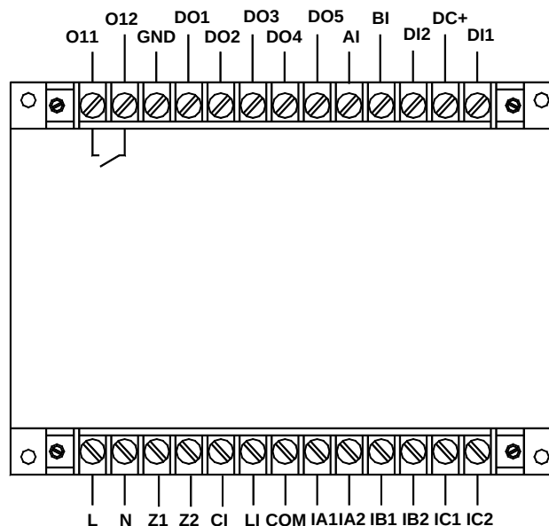
AMDG-X/E811 系列保护器主单元端子图
