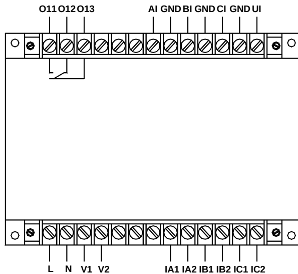
AMDG-X/F101 系列保护器主单元端子图
