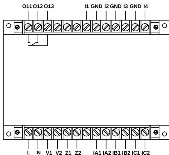
AMDG-X/F111 系列保护器主单元端子图
