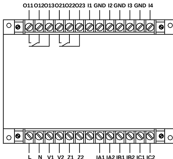
AMDG-X/F112 系列保护器主单元端子图
