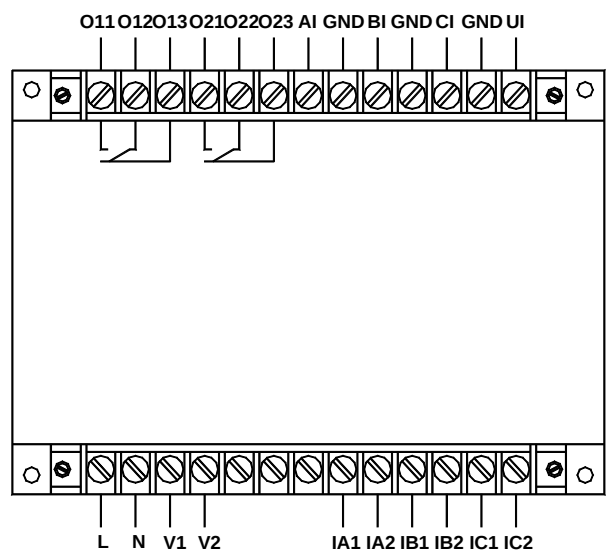
AMDG-X/F102 系列保护器主单元端子图
