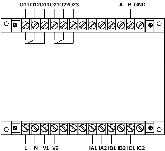
AMDG-X/F202 系列保护器主单元端子图
