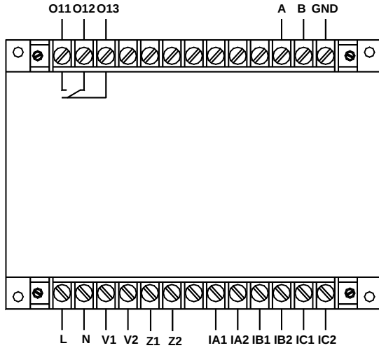
AMDG-X/F211 系列保护器主单元端子图
