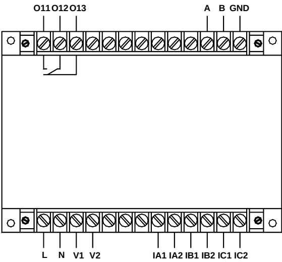
AMDG-X/F201 系列保护器主单元端子图
