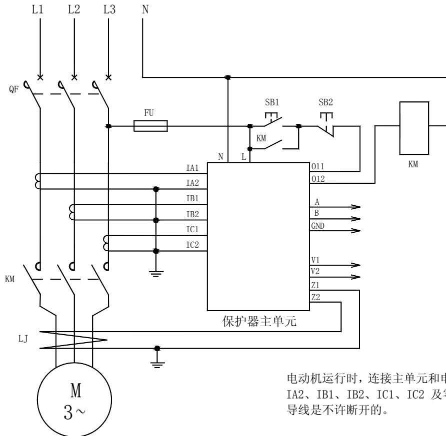
AMDG-X/F21□ 系列电动机保护器应用电气原理图
