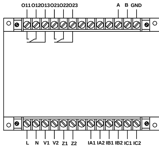
AMDG-X/F212 系列保护器主单元端子图
