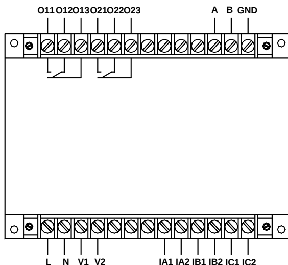
AMDG-X/F3□2 系列保护器主单元端子图
