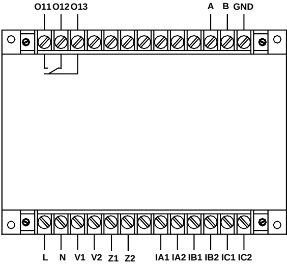
AMDG-X/F31□ 系列保护器主单元端子图
