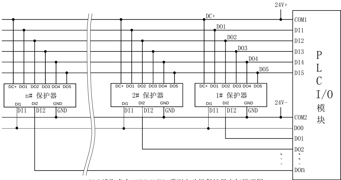
PLC 读取多台 AMDG-X/F8 系列电动机保护器电气原理图
