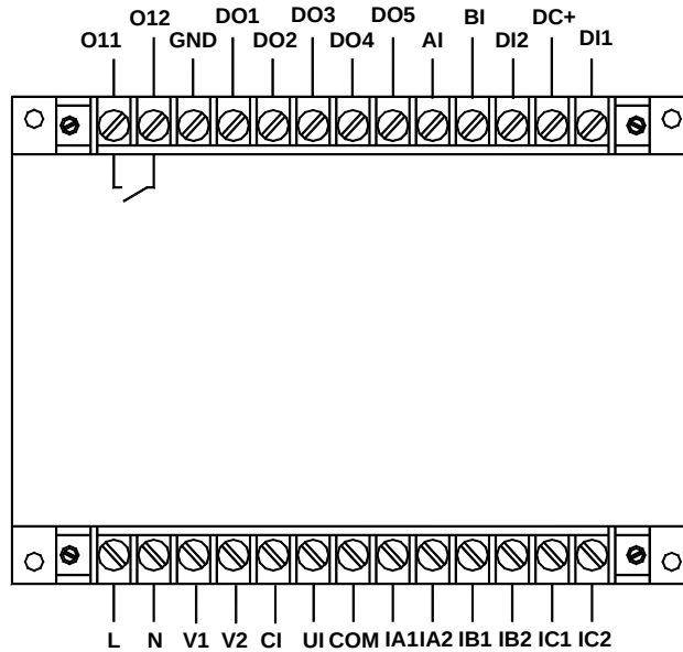
AMDG-X/F8□1 系列保护器主单元端子图
