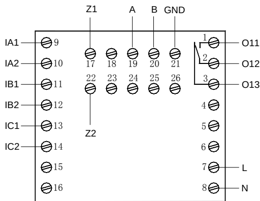
AMDP-□/C311 系列保护器主单元端子图
