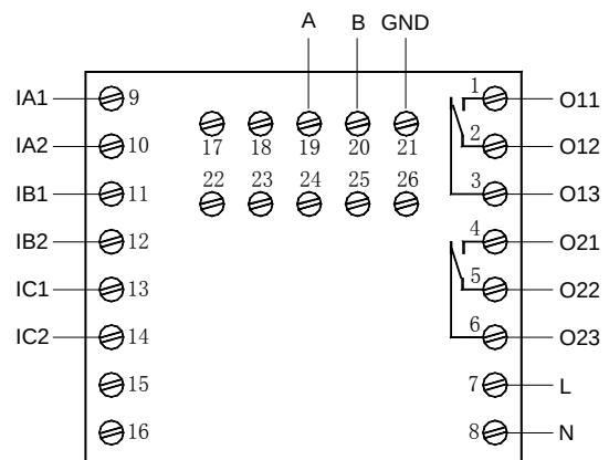
AMDP-□/C302 系列保护器主单元端子图
