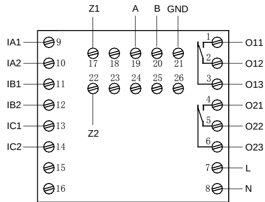
AMDP-□/C312 系列保护器主单元端子图
