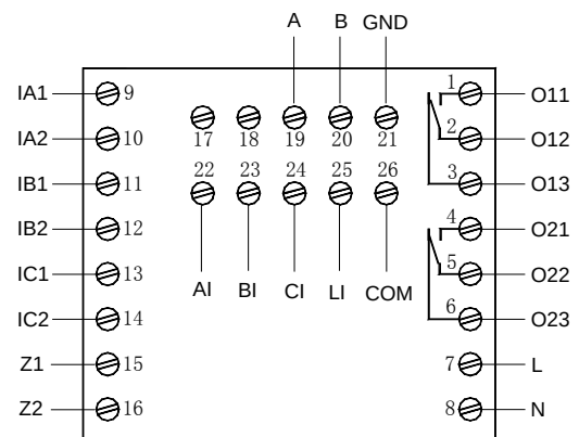
AMDP-□/C412 系列保护器主单元端子图
