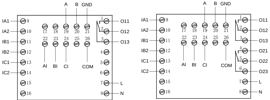
AMDP-□/C401 系列保护器主单元端子图
