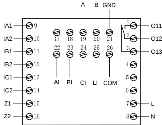
AMDP-□/C411 系列保护器主单元端子图
