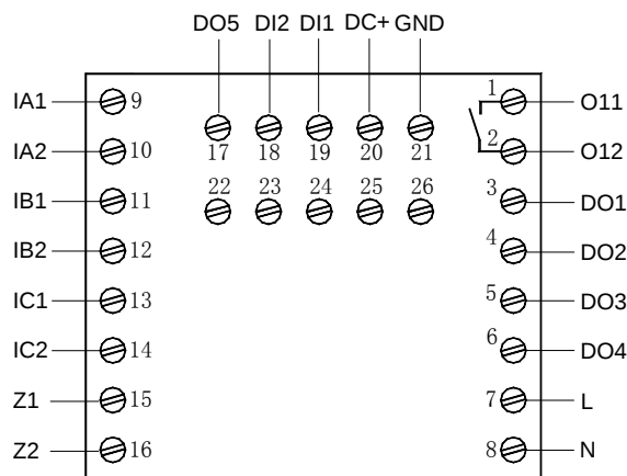
AMDP-□/C611 系列保护器主单元端子图
