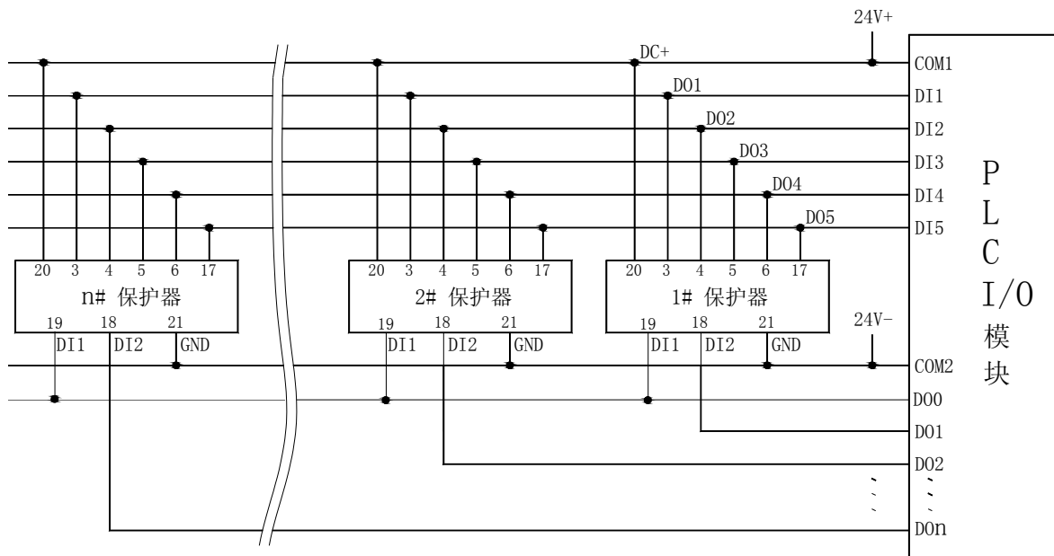
PLC 读取多台 AMDP-□/C6 系列电动机保护器电气原理图
