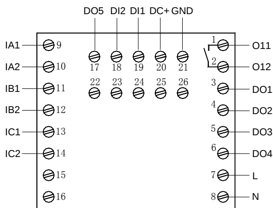
AMDP-□/C601 系列保护器主单元端子图
