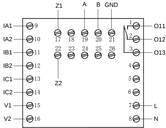
AMDP-□/D211 系列保护器主单元端子图
