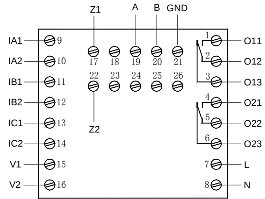
AMDP-□/D212 系列保护器主单元端子图
