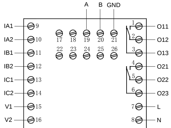
AMDP-□/D202 系列保护器主单元端子图
