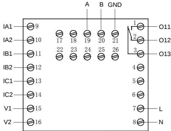
AMDP-□/D201 系列保护器主单元端子图
