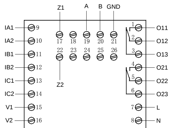
AMDP-□/D312 系列保护器主单元端子图
