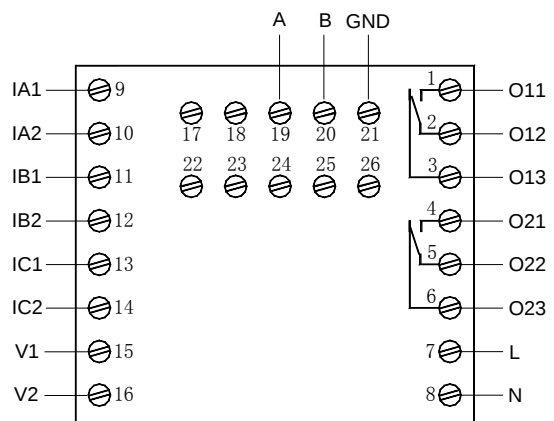
AMDP-□/D302 系列保护器主单元端子图
