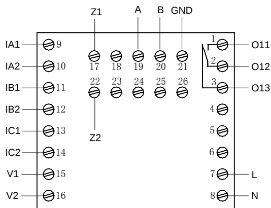
AMDP-□/D311 系列保护器主单元端子图
