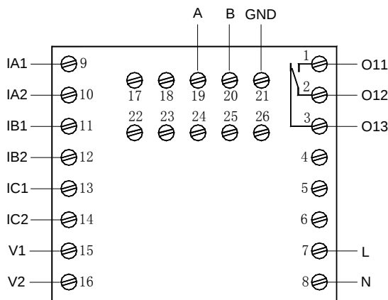
AMDP-□/D301 系列保护器主单元端子图
