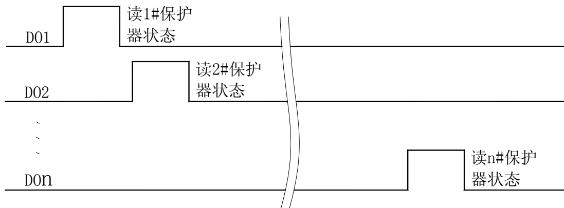
PLC 读取多台 AMDP-□/D6 系列电动机保护器时序图
