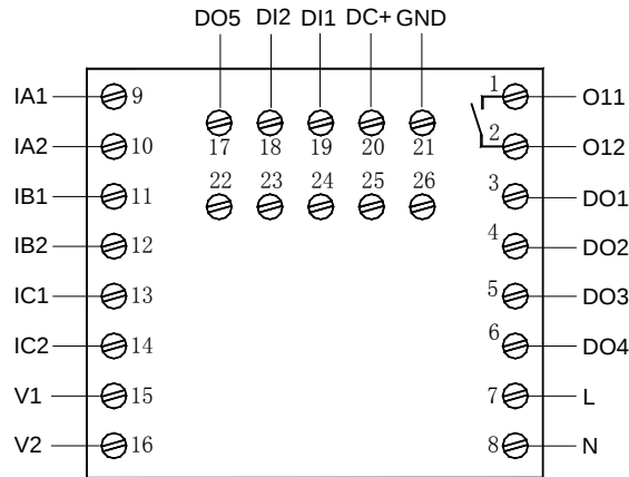
AMDP-□/D6□1 系列保护器主单元端子图
