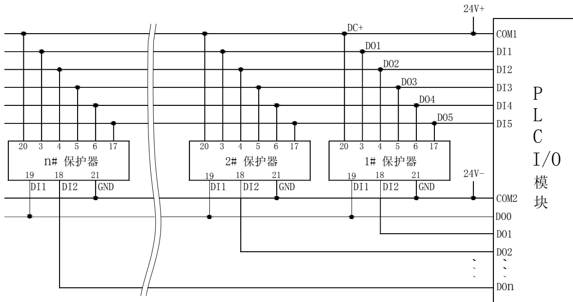
PLC 读取多台 AMDP-□/D6 系列电动机保护器电气原理图
