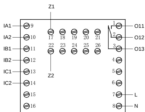
AMDP-X/E011 系列保护器主单元端子图
