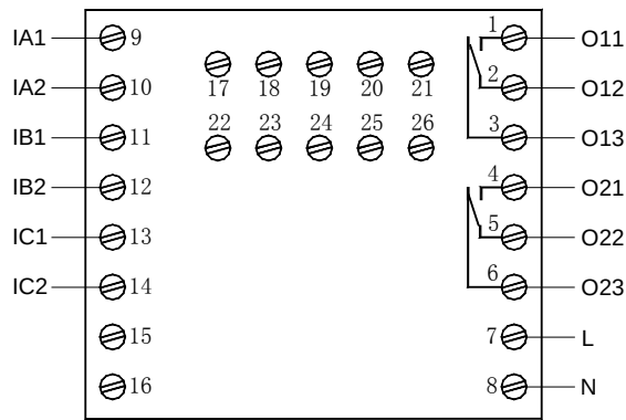
AMDP-X/E002 系列保护器主单元端子图
