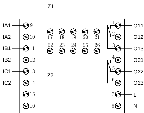
AMDP-X/E012 系列保护器主单元端子图
