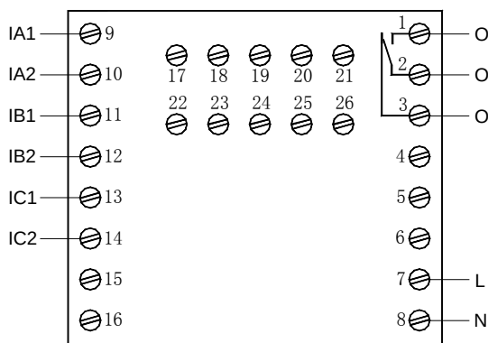
AMDP-X/E001 系列保护器主单元端子图
