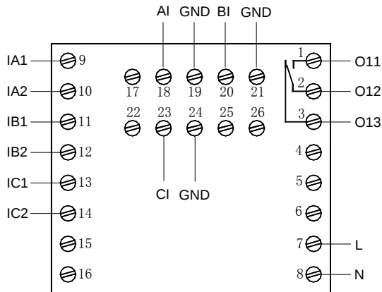
AMDP-X/E101 系列保护器主单元端子图
