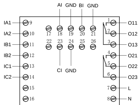
AMDP-X/E102 系列保护器主单元端子图
