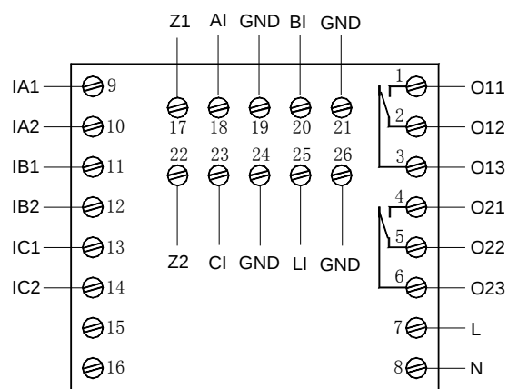
AMDP-X/E112 系列保护器主单元端子图
