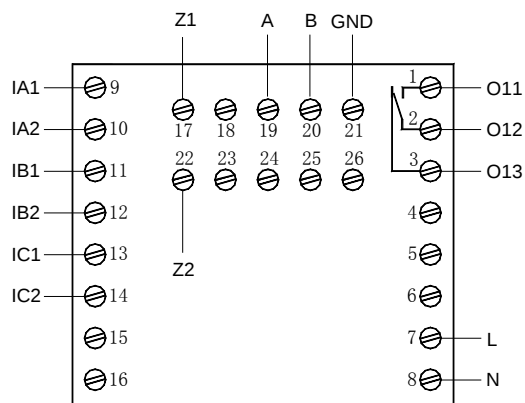
AMDP-X/E211 系列保护器主单元端子图
