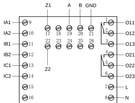
AMDP-X/E212 系列保护器主单元端子图
