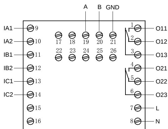
AMDP-X/E202 系列保护器主单元端子图
