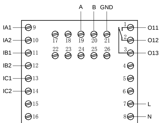
AMDP-X/E201 系列保护器主单元端子图
