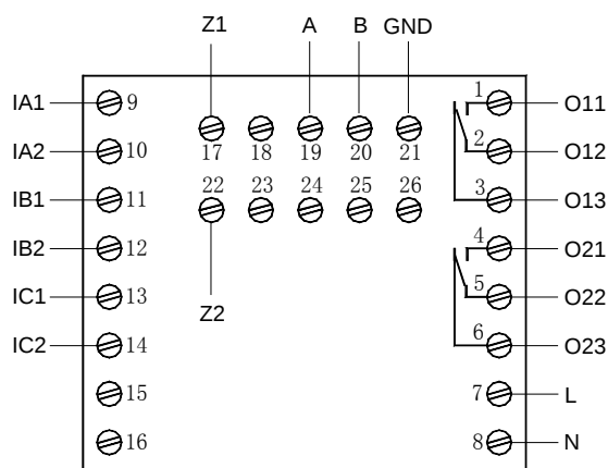
AMDP-X/E312 系列保护器主单元端子图
