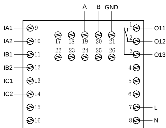
AMDP-X/E301 系列保护器主单元端子图
