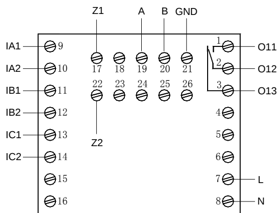
AMDP-X/E311 系列保护器主单元端子图
