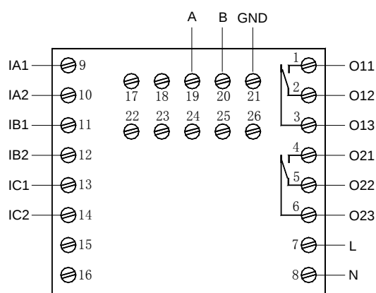
AMDP-X/E302 系列保护器主单元端子图
