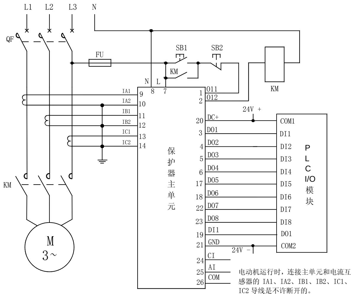
AMPD-X/E701 系列电动机保护器 D0 连接 PLC 电气原理图
