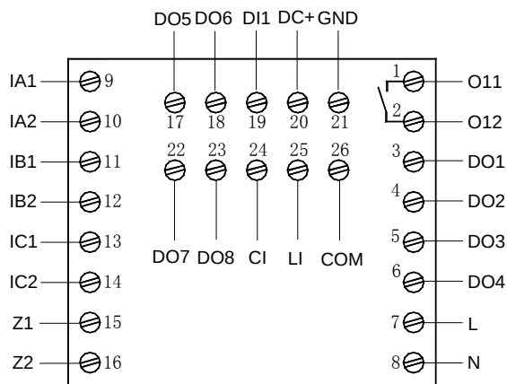
AMDP-X/E711 系列保护器主单元端子图
