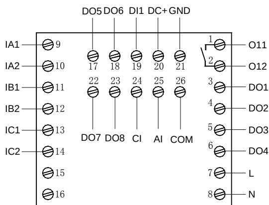
AMDP-X/E701 系列保护器主单元端子图
