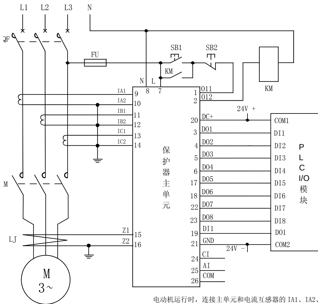
AMDP-X/E711 系列电动机保护器 D0 连接 PLC 电气原理图
