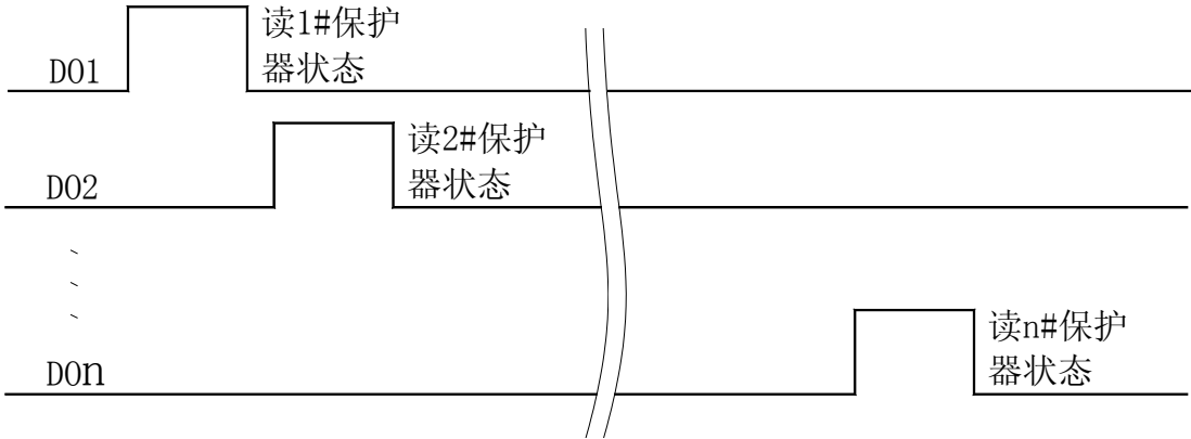
PLC 读取多台 AMDP-X/E8 系列电动机保护器时序图
