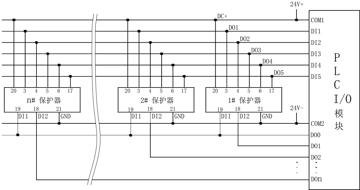
PLC 读取多台 AMDP-X/E8 系列电动机保护器电气原理图
