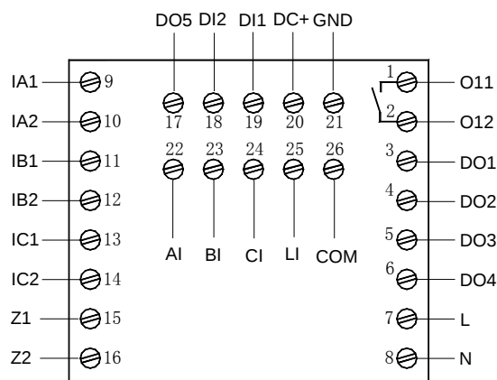
AMDP-X/E811 系列保护器主单元端子图
