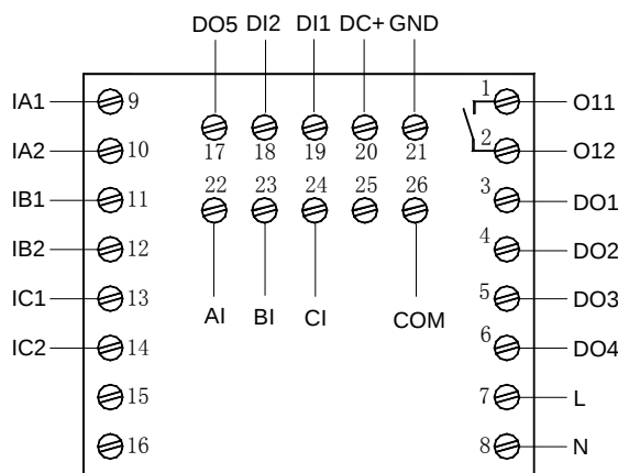
AMDP-X/E801 系列保护器主单元端子图
