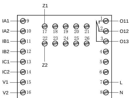
AMDP-X/F011 系列保护器主单元端子图
