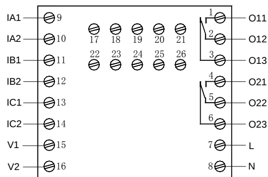
AMDP-X/F002 系列保护器主单元端子图
