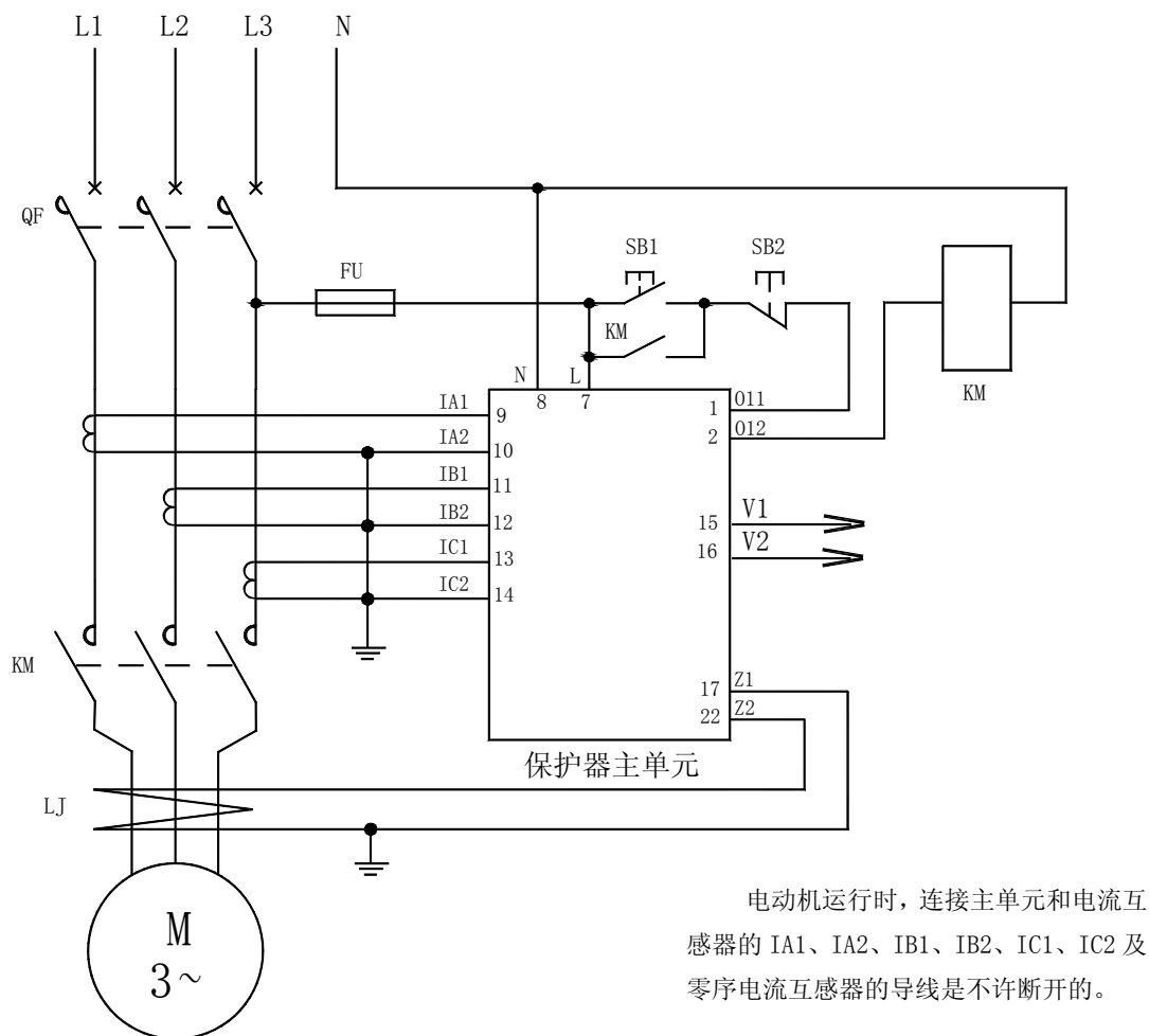
AMDP-X/F01□ 系列电动机保护器应用电气原理图
