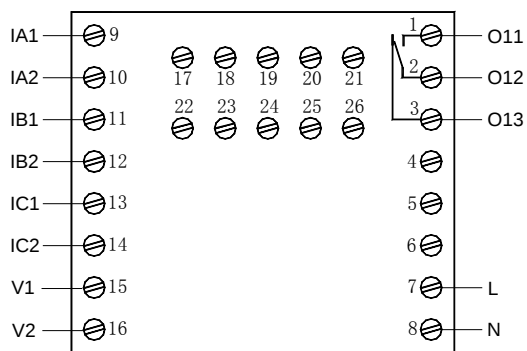
AMDP-X/F001 系列保护器主单元端子图
