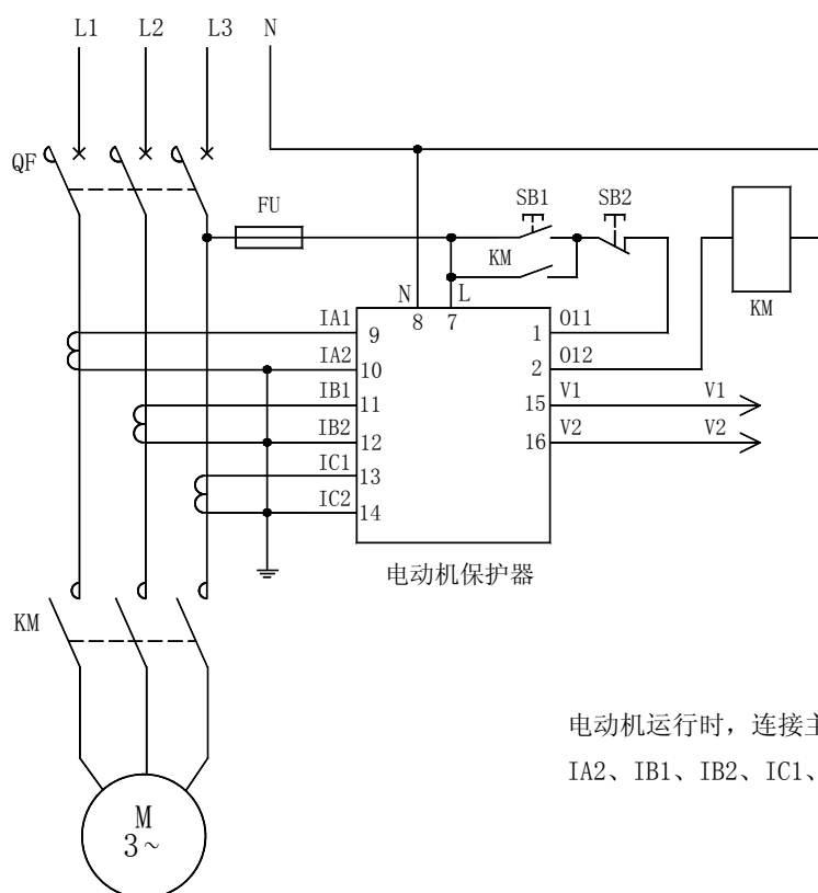
AMDP-X/F001 系列保护器主单元端子图
