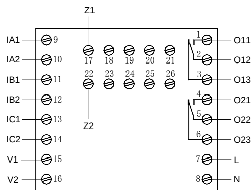
AMDP-X/F012 系列保护器主单元端子图
