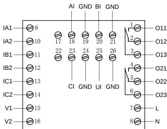
AMDP-X/F102 系列保护器主单元端子图
