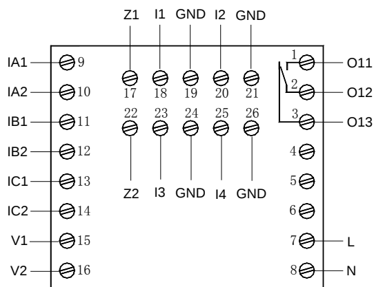
AMDP-X/F111 系列保护器主单元端子图
