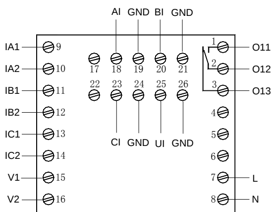
AMDP-X/F101 系列保护器主单元端子图
