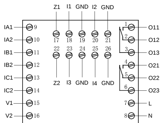
AMDP-X/F112 系列保护器主单元端子图
