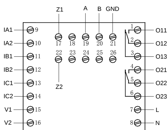
AMDP-X/F212 系列保护器主单元端子图
