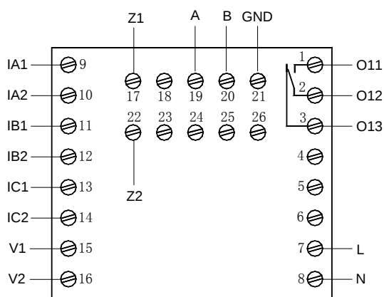
AMDP-X/F211 系列保护器主单元端子图
