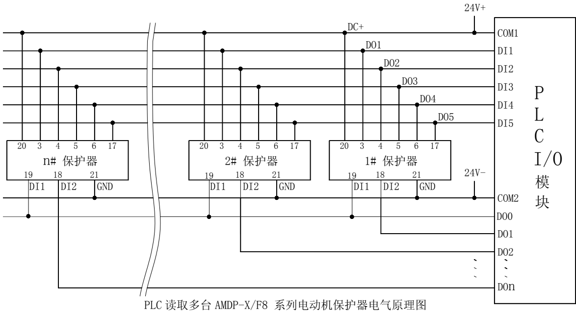
PLC 读取多台 AMDP-X/F8 系列电动机保护器电气原理图
