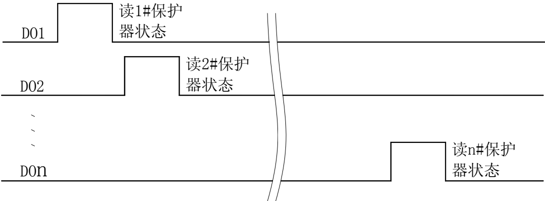
PLC 读取多台 AMDP-X/F8 系列电动机保护器时序图
