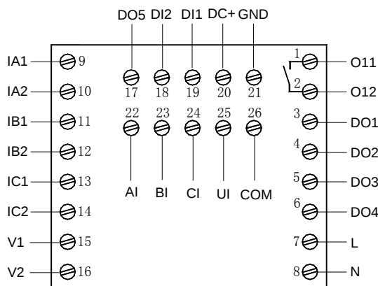
AMDP-X/F8□1 系列保护器主单元端子图
