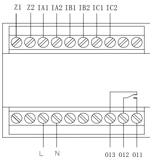
AMDS-□/B011 系列保护器主单元端子图
