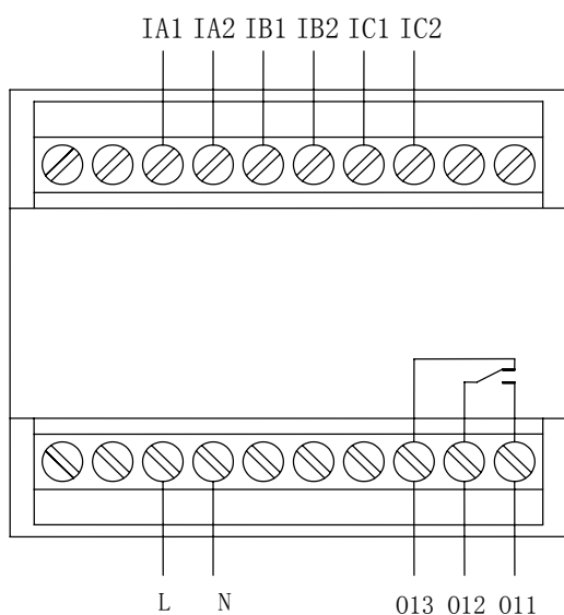
AMDS-□/B001 系列保护器主单元端子图
