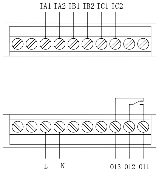
AMDS-□/D001、AMDS-□/D021 主单元端子图 AMDS-□/D031、AMDS-□/D041 主单元端子图
