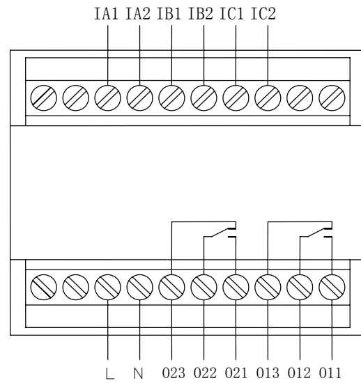
AMDS-□/D002、AMDS-□/D022 主单元端子图 AMDS-□/D032、AMDS-□/D042 主单元端子图
