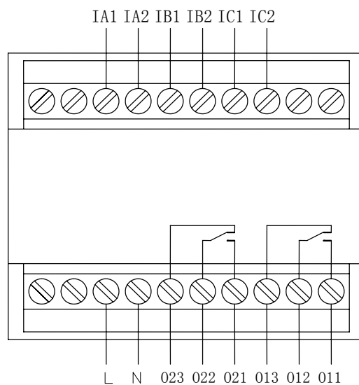
AMDS-X/E002 主单元端子图
