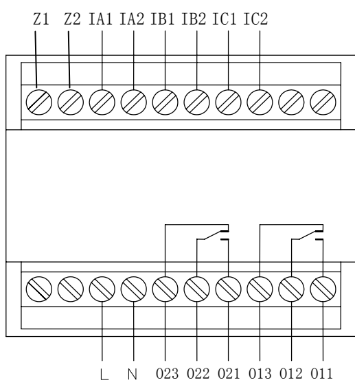
AMDS-X/E012 主单元端子图
