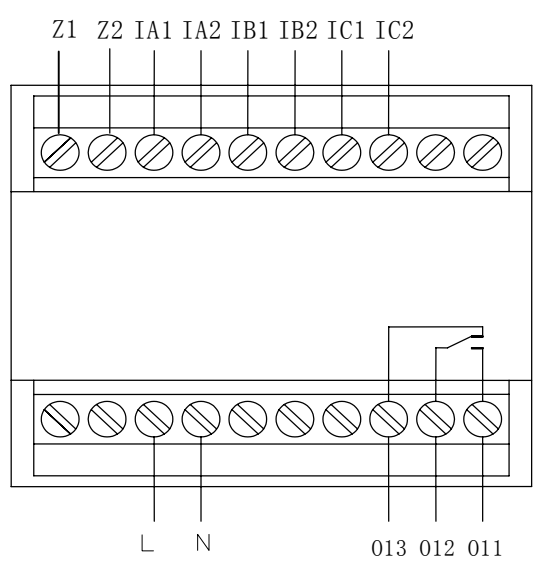
AMDS-X/E011 主单元端子图
