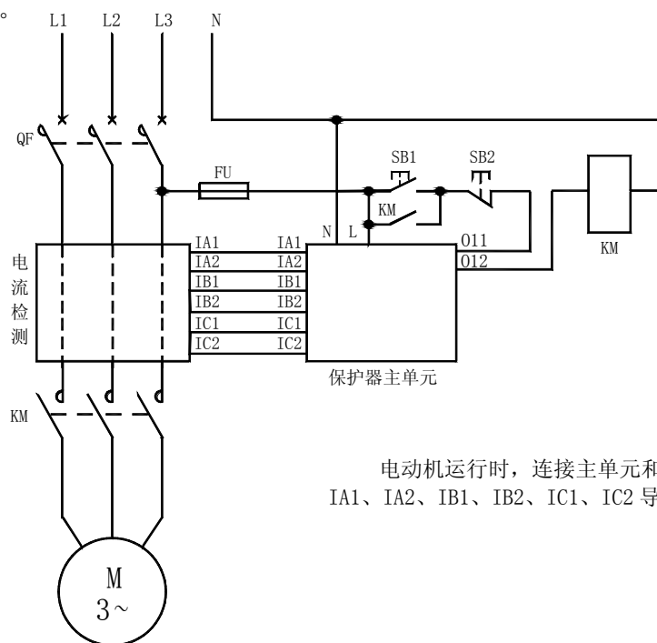
AMDG-□/CO 系列电动机保护器应用电气原理图
