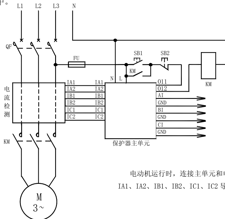
AMDG-□/C1 系列电动机保护器应用电气原理图
