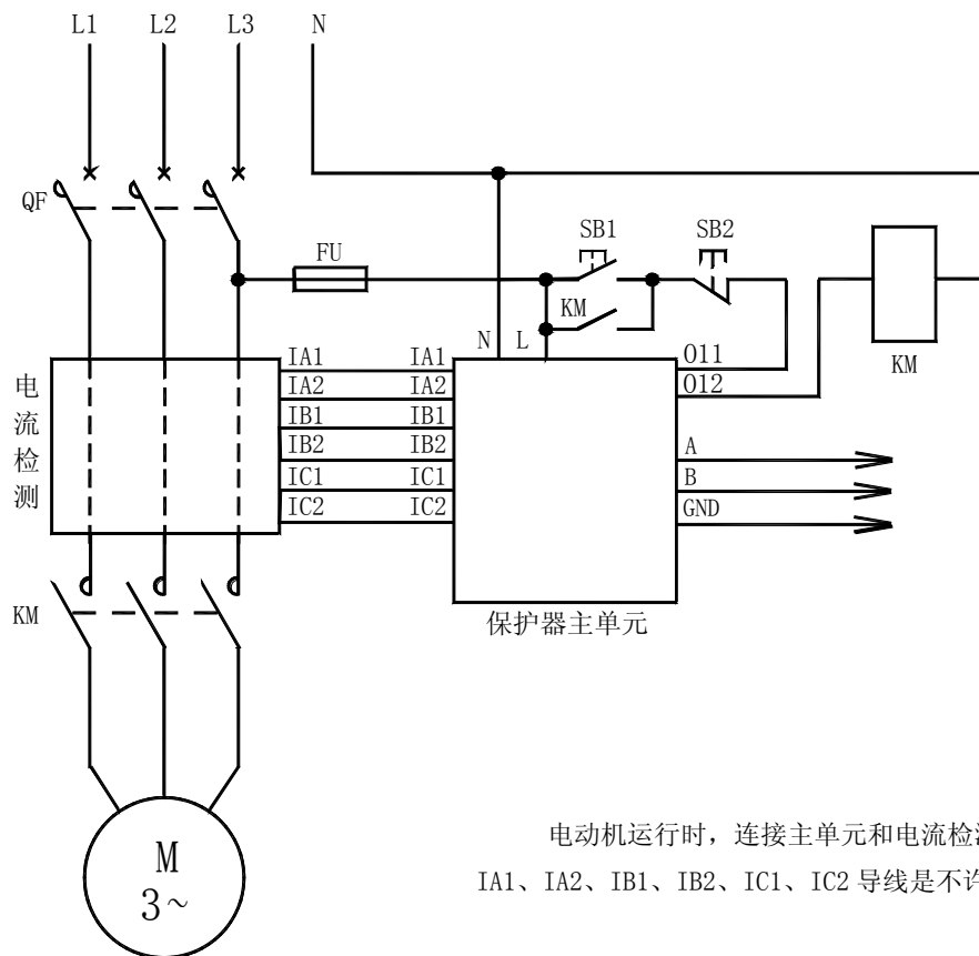
AMDG-□/C2 系列电动机保护器应用电气原理图
