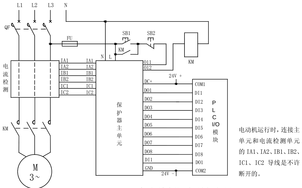
AMDG-□/□/C5 系列电动机保护器应用电气原理图
