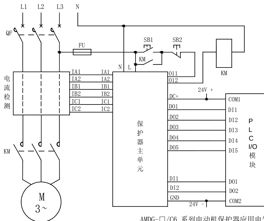
AMDG-□/C6 系列电动机保护器应用电气原理图
