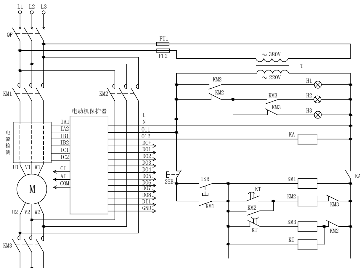
图 2 电动机保护器用于星/三角起动 (检测线电流) 电气原理图
