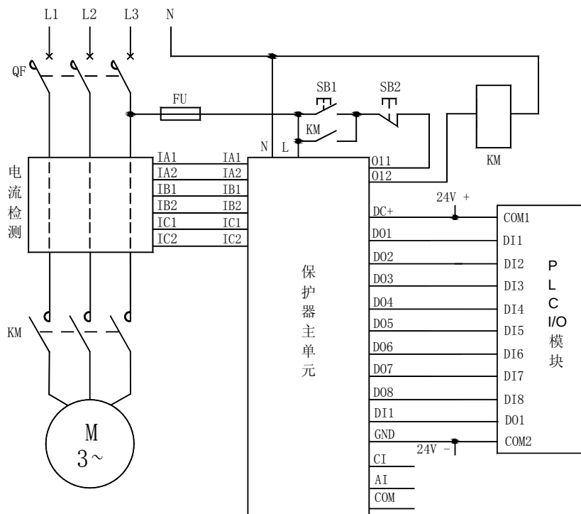
AMDG-□/C7 系列电动机保护器应用电气原理图
