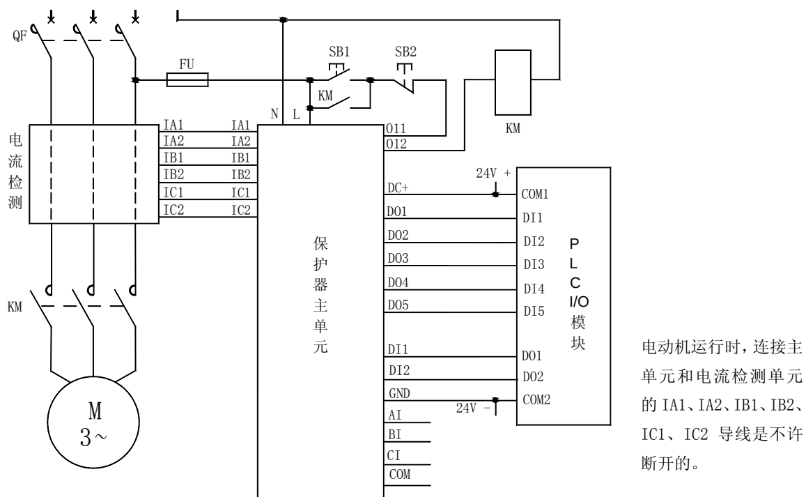
AMDG-□/C8 系列电动机保护器应用电气原理图
