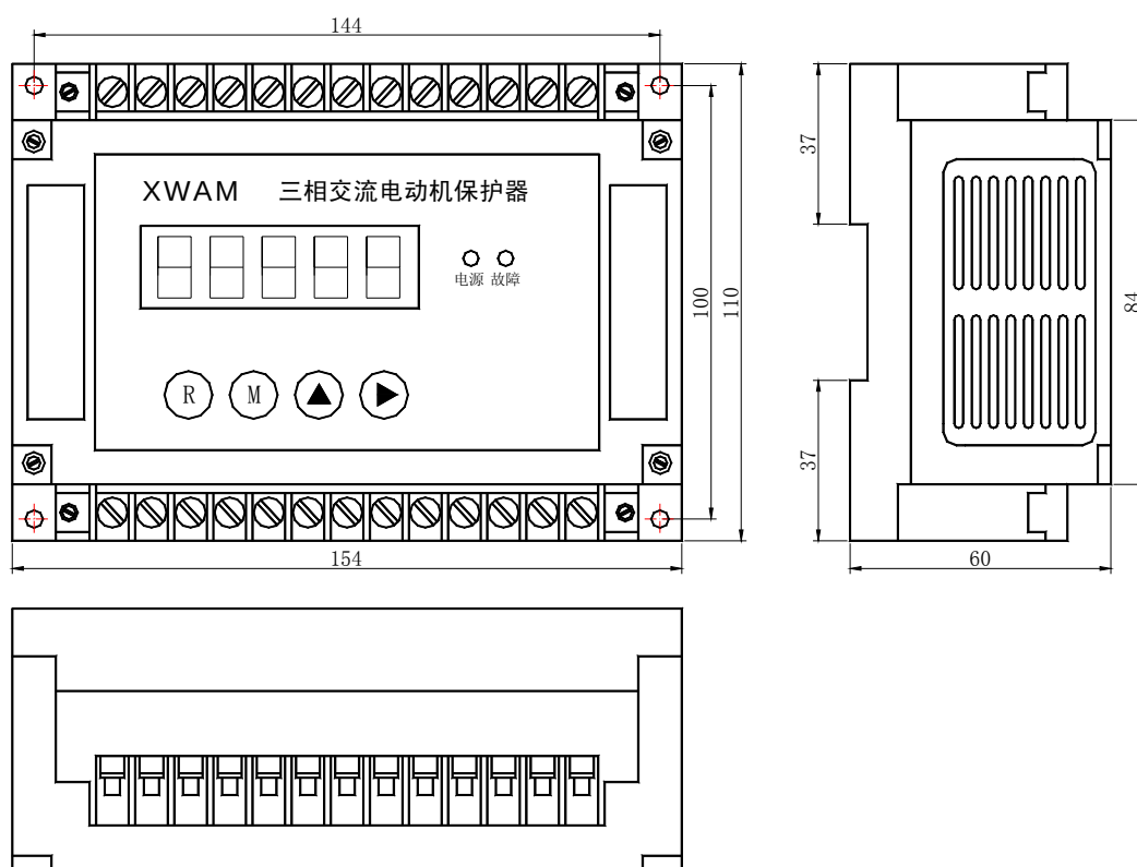
AMDG-□/C8 系列电动机保护器主单元外形及安装孔尺寸
