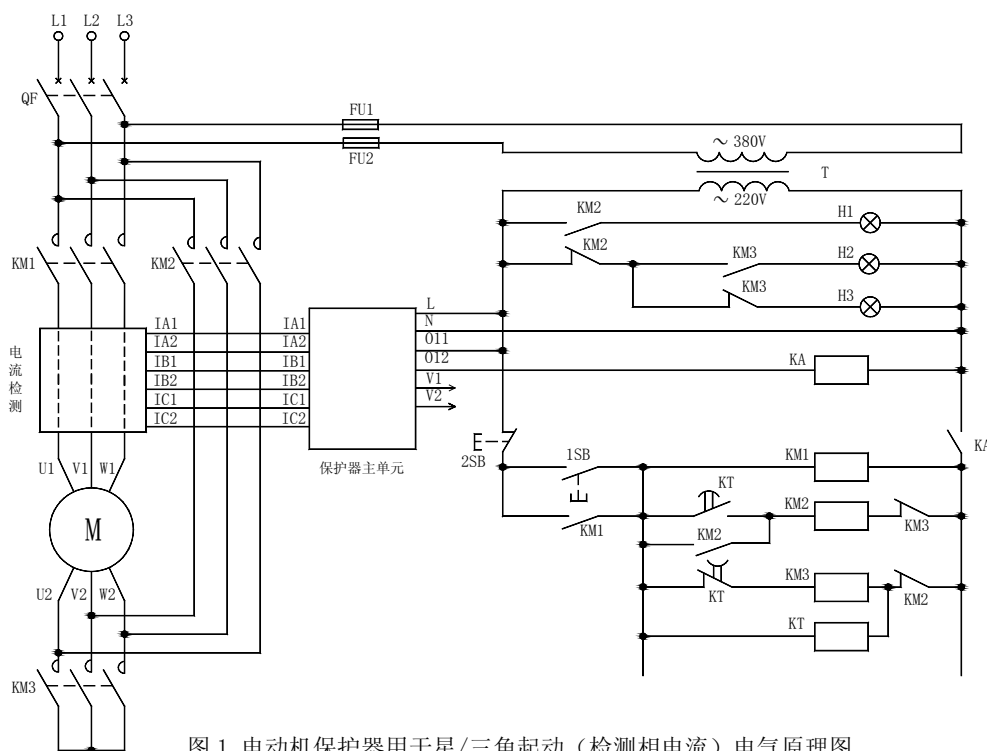
图 1 电动机保护器用于星/三角启动（检测相电流）电气原理图
