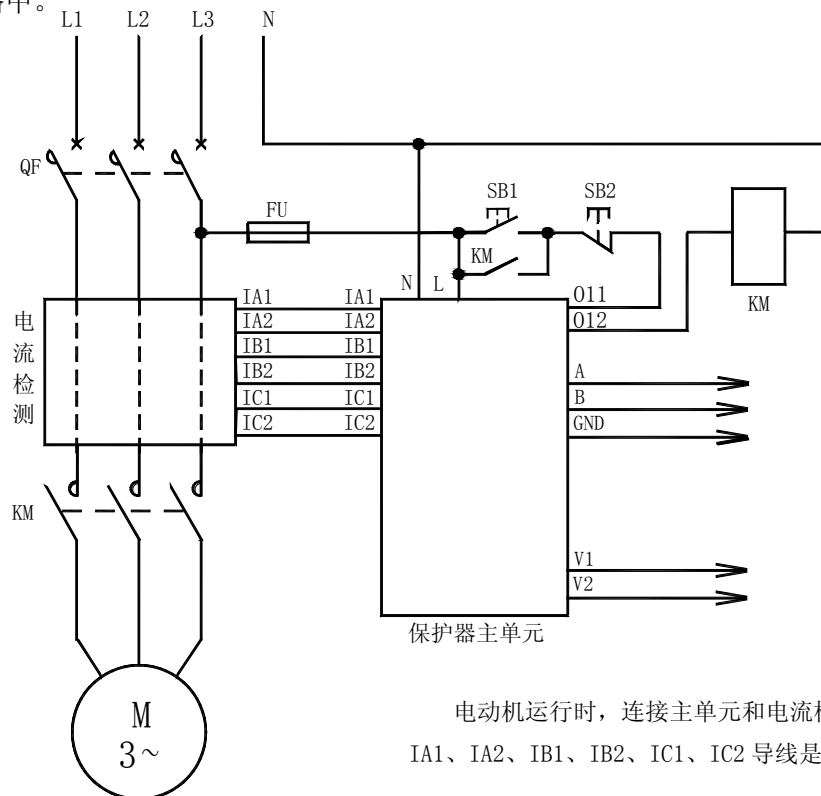
AMDG-□/D2 系列电动机保护器应用电气原理图
