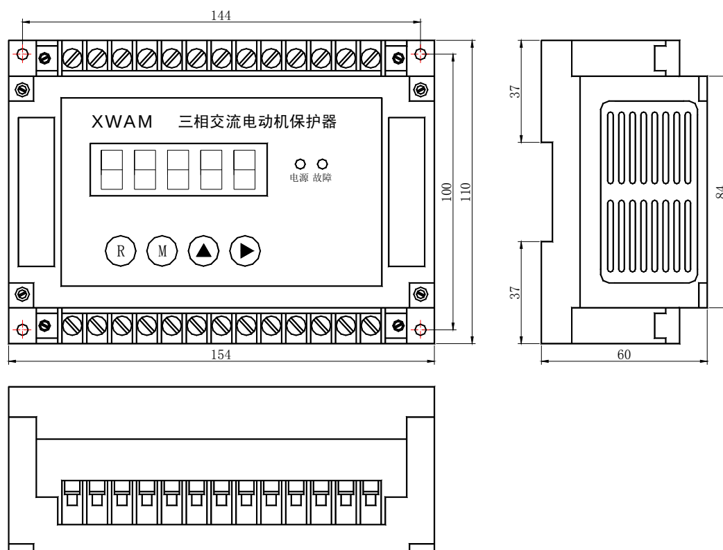
AMDG-□/D5 系列电动机保护器主单元外形及安装孔尺寸
