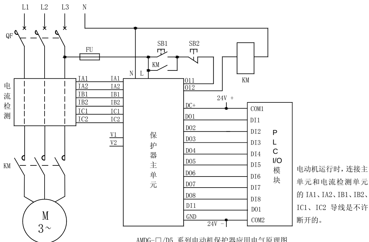
AMDG-□/D5 系列电动机保护器应用电气原理图
